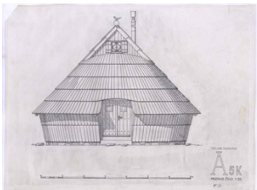
Vlasto Kopač, Velika planina, A5K, prednje čelo in prečni rez, 1 : 20, črnilo na transparentnem papirju, hrani MAO
