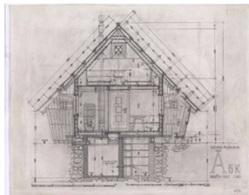
Vlasto Kopač, Velika planina, A5K, prednje čelo in prečni rez, 1 : 20, črnilo na transparentnem papirju, hrani MAO
